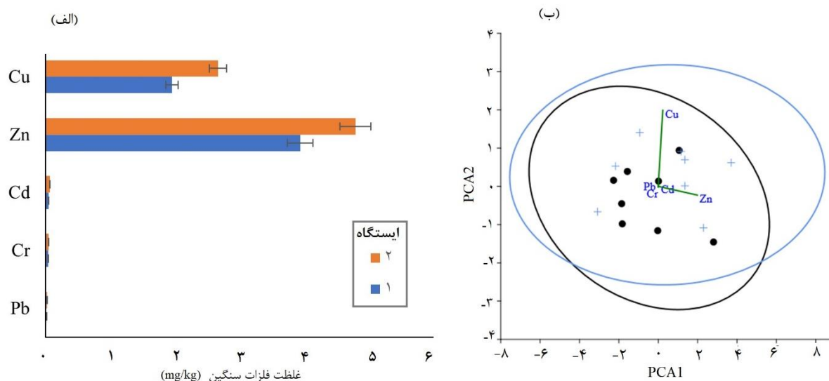
شکل ۲. مقایسه گرافیکی غلظت فلزات سنگین بر اساس نتایج آزمون کرومکال-والیس (الف) و چند متغیره مولفه‌های اصلی (PCA) با استفاده از دو مولفه اصلی اول (PCs) (ب) در سیاه ماهی هراتی ( C. aculeata ) از دو ایستگاه نمونه‌برداری در رودخانه قره جای استان مرکزی
