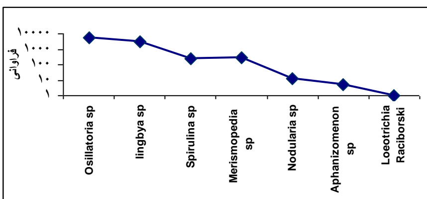
شکل ۶: فراوانی گونه های سیانوباکتری های (در مقیاس لگاریتمی) بخش جنوبی دریای خزر (تنکابن-امیرآباد) در پاییز ۱۳۸۸
