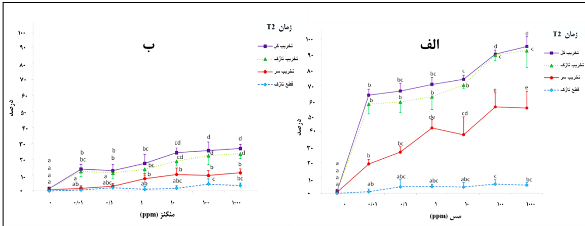
شکل ۴: نمودار درصد تخریب اسپیرم مارماهی دهان‌گرد خزری ( Caspiomyzon wagneri ).
