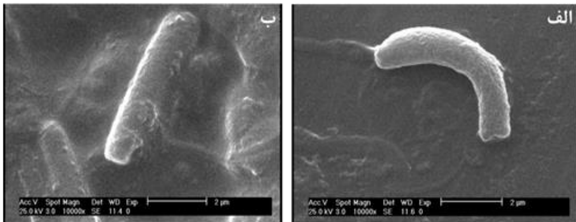
شکل ۵: (الف) تخریب دیواره‌ی سلولی در اسپیرم مارماهی دهان‌گرد خزری ( Caspiomyzon wagneri ). تحت تأثیر ۱۰۰ میلی‌گرم در لیتر منگنز به مدت سه ساعت (ب) اسپیرم مارماهی دهان‌گرد خزری در تماس با غلظت ۱۰ میلی‌گرم در لیتر مس در زمان ۳۶ ساعت. میکروسکوپ الکترونی (۱۰۰۰۰X).
