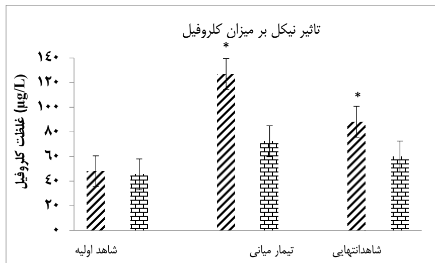
شکل ۱: مقایسه محتوای کلروفیل، بین تیمار فلز نیکل و شاهد در جمعیت جلبک سبز Nannochloropsis oculata
