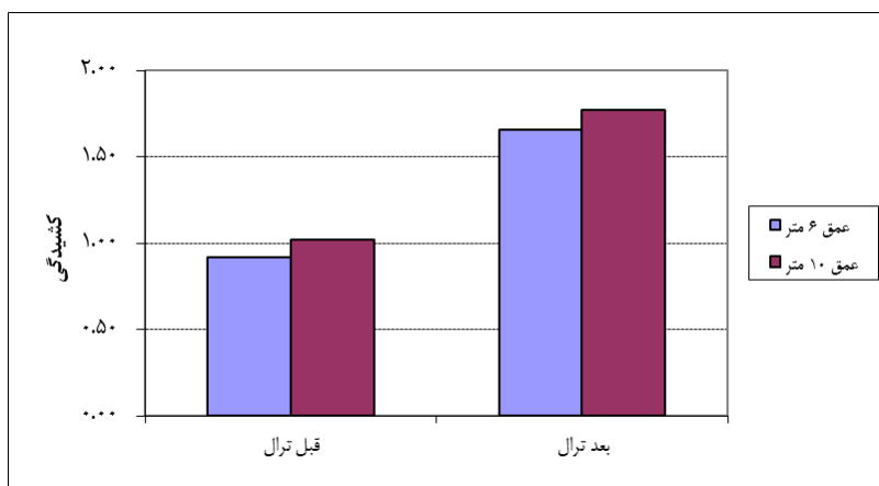
شکل 5: مقدار کشیده گی در مقیاس Ø در منطقه بحرکان در سال ۱۳۸۹
