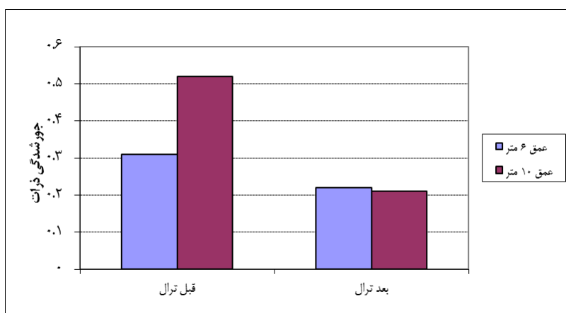
شکل 6: جورشدگی ذرات در مقیاس Ø در منطقه بحرکان در سال ۱۳۸۹
