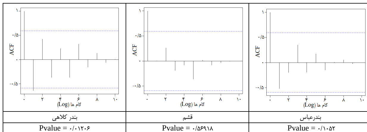
شکل ۸: نمودار خطاهای پیش‌بینی میزان CPUE (کیلوگرم بر شناور روز) میگوی سر تیز ( Metapenaeus affinis ) در مناطق بندرعباس، قشم و بندر کلاهی برای سال‌های ۱۳۹۹ تا ۱۴۰۳.
