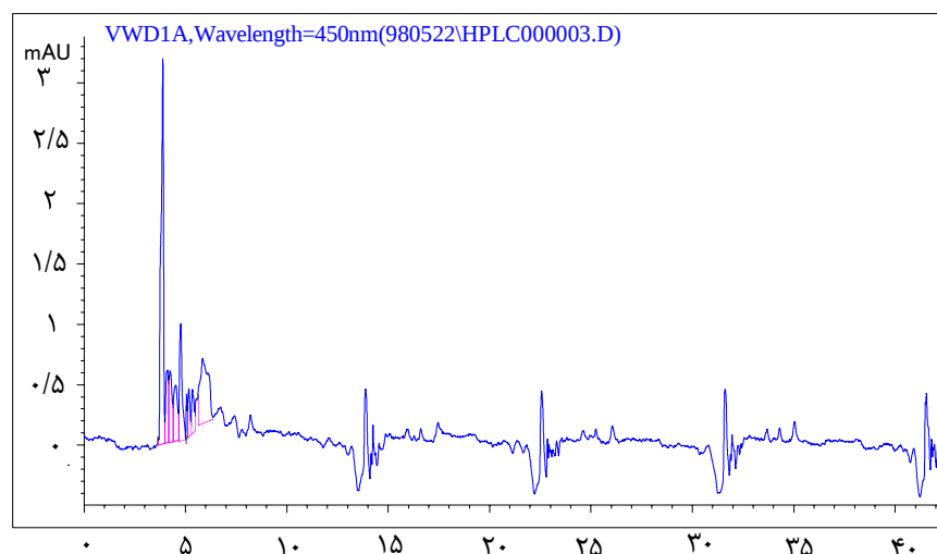
شکل ۲: کروماتوگرام HPLC فوکوزانتین (پیک حضور فوکوزانتین {RetTime} در دقیقه ۳٫۹۸ برای نمونه استخراج شده از جلبک قهوه‌ای Colpomenia sinuosa (سواحل جزیره قشم، ۱۳۹۷).
