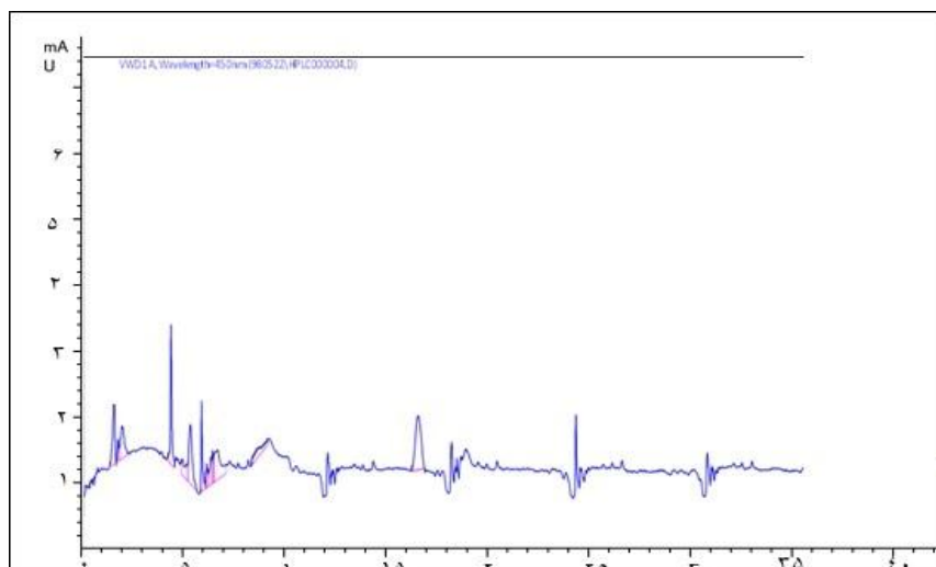
شکل ۱: کروماتوگرام HPLC فوکوزانتین استاندارد (پیک حضور فوکوزانتین {RetTime} در دقیقه ۴٫۶۰ برای استاندارد) (سواحل جزیره قشم، ۱۳۹۷).
