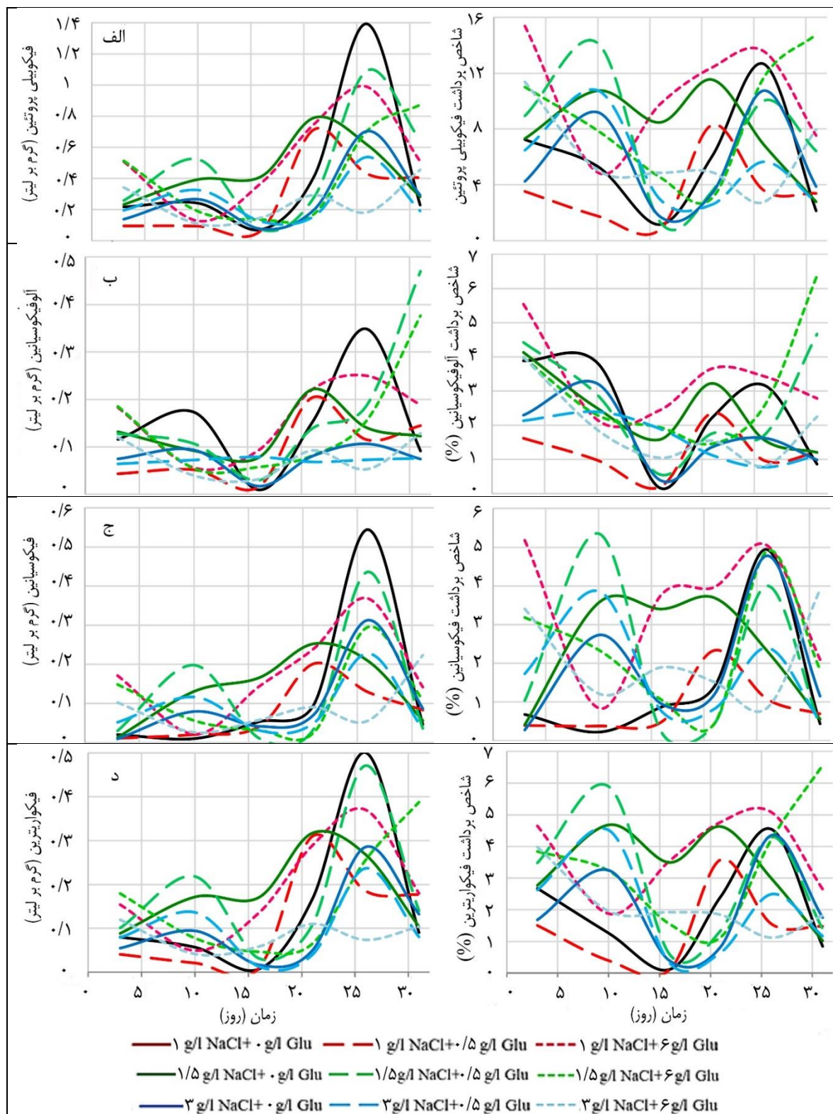
شکل ۳: میزان و شاخص برداشت الف. فیکوبیلی پروتئین‌ها، ب. آلفیکوسیانین، ج. فیکوسیانین و د. فیکواریترین.
