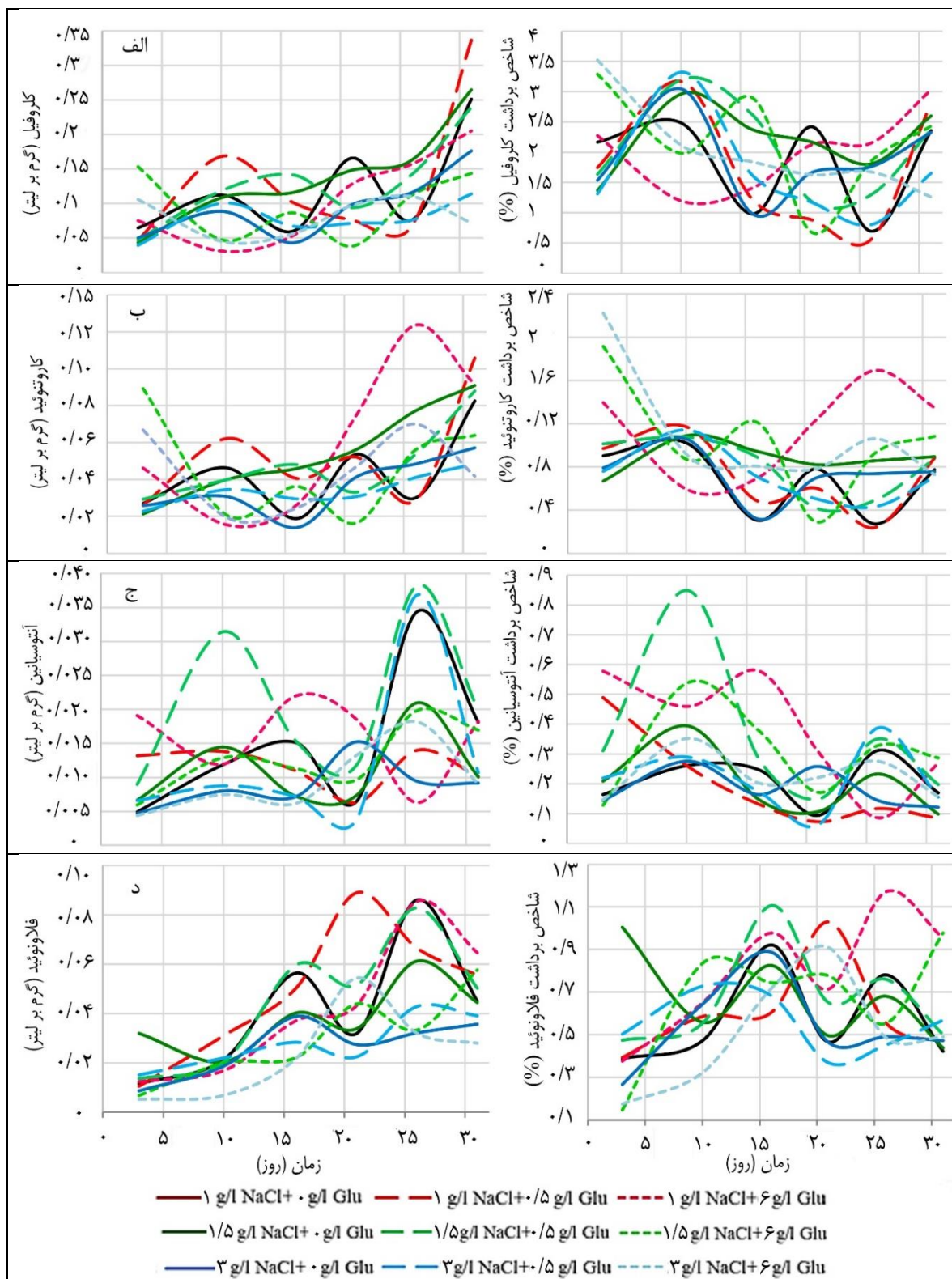
شکل ۲: میزان و شاخص برداشت الف. کلروفیل آ، ب. کارتنوئیدها، ج. آنتوسیانین، د. فلاونوئید.
