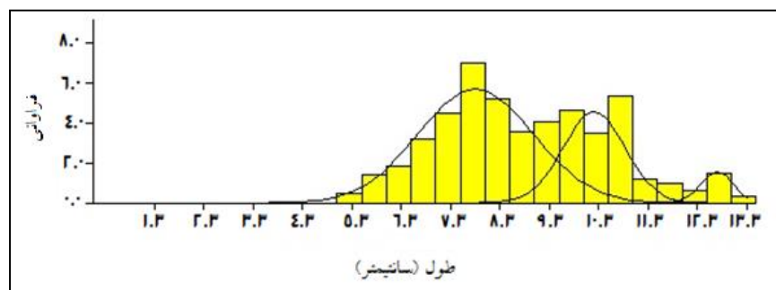
شکل ۱۱: نمودار توزیع فراوانی طولی گروه‌های همزاد جداسازی شده گونه آترین ماهی دریای خزر ( Atherina caspia ) برای جنس ماده در خلیج گرگان-جنوب شرق دریای خزر (۱۳۹۵-۱۳۹۶).
