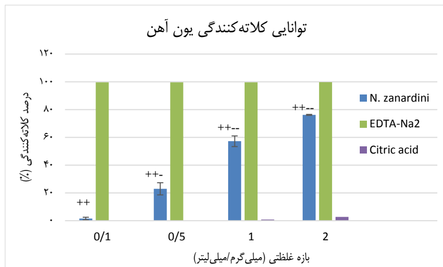
شکل ۱: توانایی کلیت‌کنندگی یون آهن توسط عصاره آبی جلبک Nizimuddinina zanardini .
