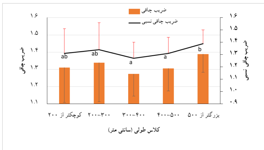
شکل ۲: میانگین ( \pm انحراف معیار) ضریب چاقی و ضریب چاقی نسبی ماهی سفید در کلاس طولی مختلف و مقایسه آن‌ها در منطقه جنوب شرقی دریای خزر (گهرباران).
