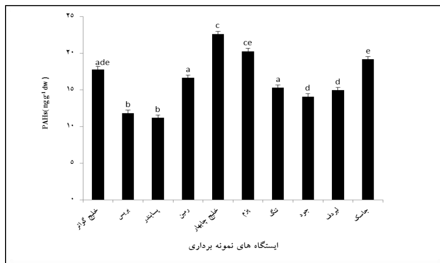
شکل ۲: مجموع ترکیبات هیدروکربن‌های آروماتیک چند حلقه‌ای در بافت خرچنگ منزوی ( Clibanarius signatus ) در ایستگاه‌های مختلف نمونه‌برداری (پاییز ۱۳۹۶).
