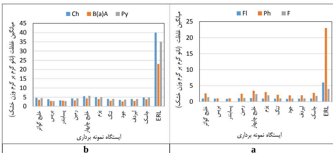
شکل ۵: (a) مقایسه غلظت ترکیبات فلورن (F) فنانترن (Ph) و فلورانتن (Fl) با میزان ERL و (b) مقایسه غلظت ترکیبات پایرن (Py)، بنزوای آنتراسن (B(a)A) و کرایسن (Ch) با میزان ERL در بافت خرچنگ منزوی ( Clibanarius signatus ) (پاییز ۱۳۹۶).
