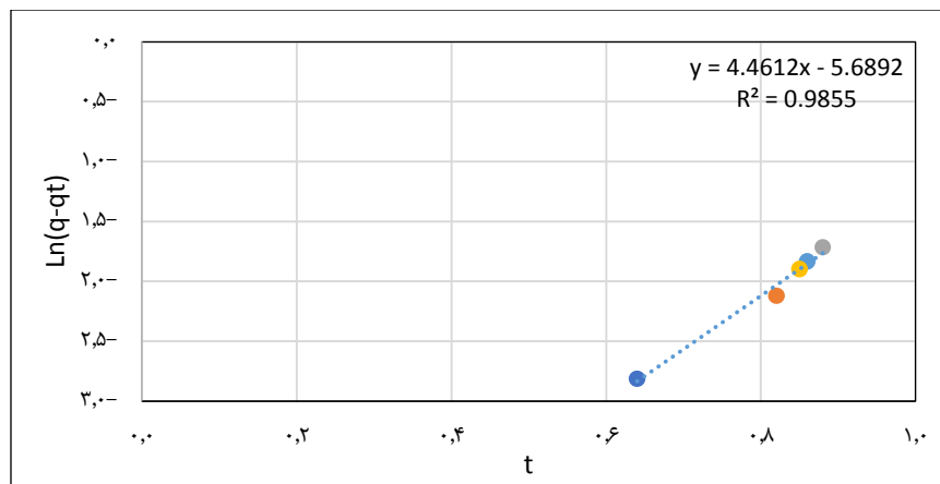
شکل ۹: رسم خطی معادله لاگرن در جذب کادمیوم توسط جلبک Scenedesmus sp.
