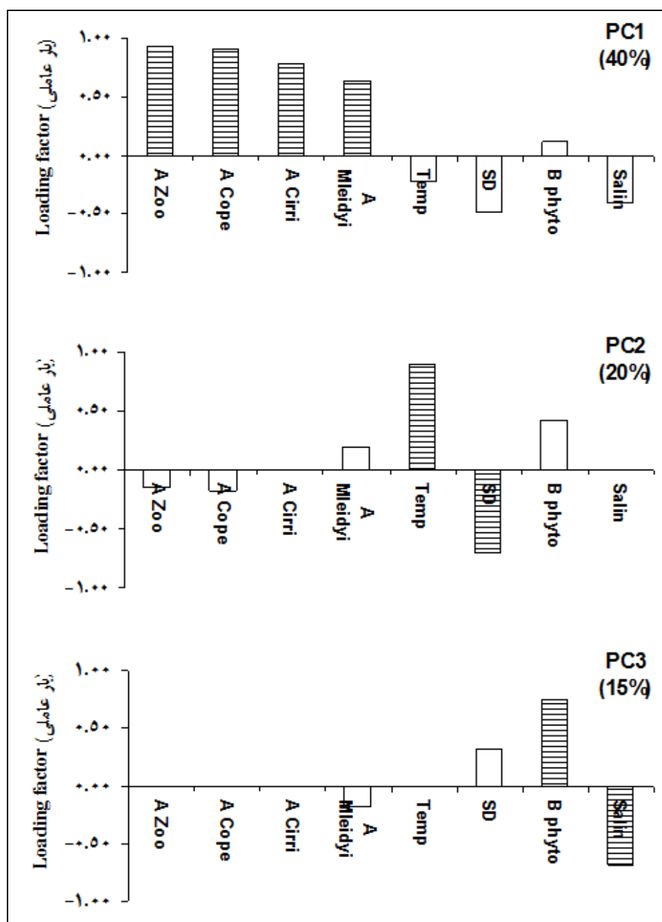
شکل ۴: تغییرات بار عاملی سه مولفه اصلی در آزمون PCA در فصل تابستان حوزه جنوبی دریای خزر (سال ۱۳۸۸) (بار عاملی بالاتر از ۰/۶۰ با ستون‌های راه نشان داده شد). علائم اختصاری نظیر جدول ۳ می باشد.
