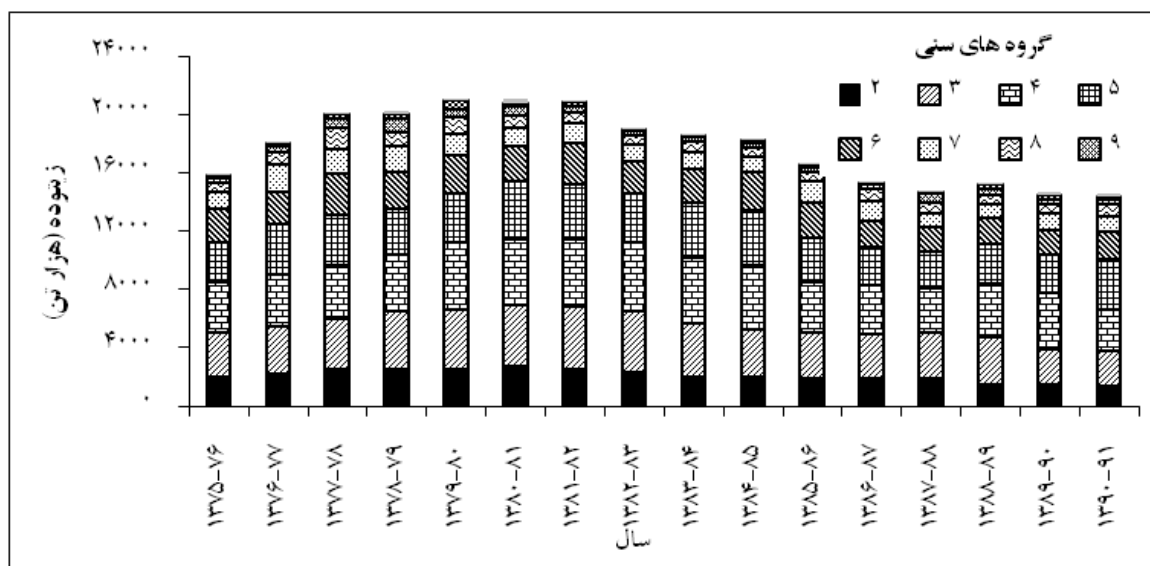
شکل ۵: مقدار ذخایر در سنین مختلف ماهی کفال طلایی در سواحل ایرانی دریای خزر طی سال‌های بهره‌برداری ۷۶-۷۵ الی ۱۳۷۵-۱۳۹۱.
